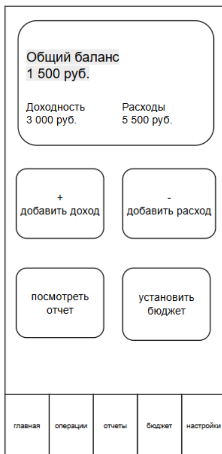
Рисунок 3.4 – Макет интерфейса главного экрана
