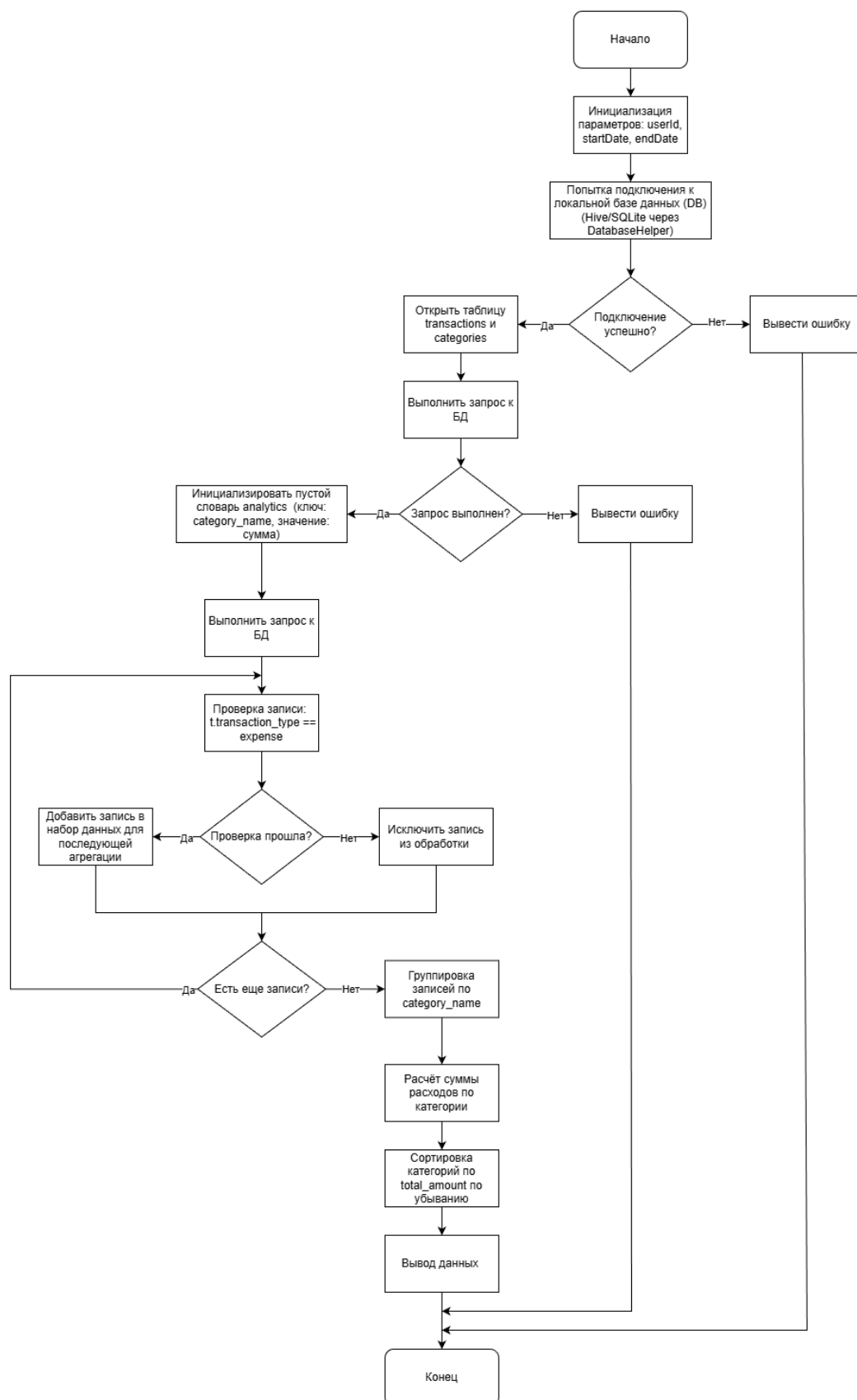
Рисунок 3.2 – Алгоритм агрегации по категориям
