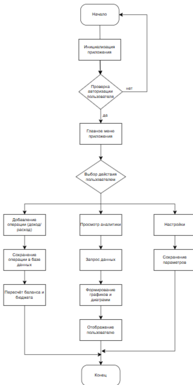
Рисунок 3.1 – Общий алгоритм работы приложения
