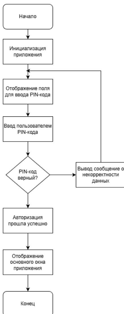
Рисунок 3.2 – Алгоритм авторизации
